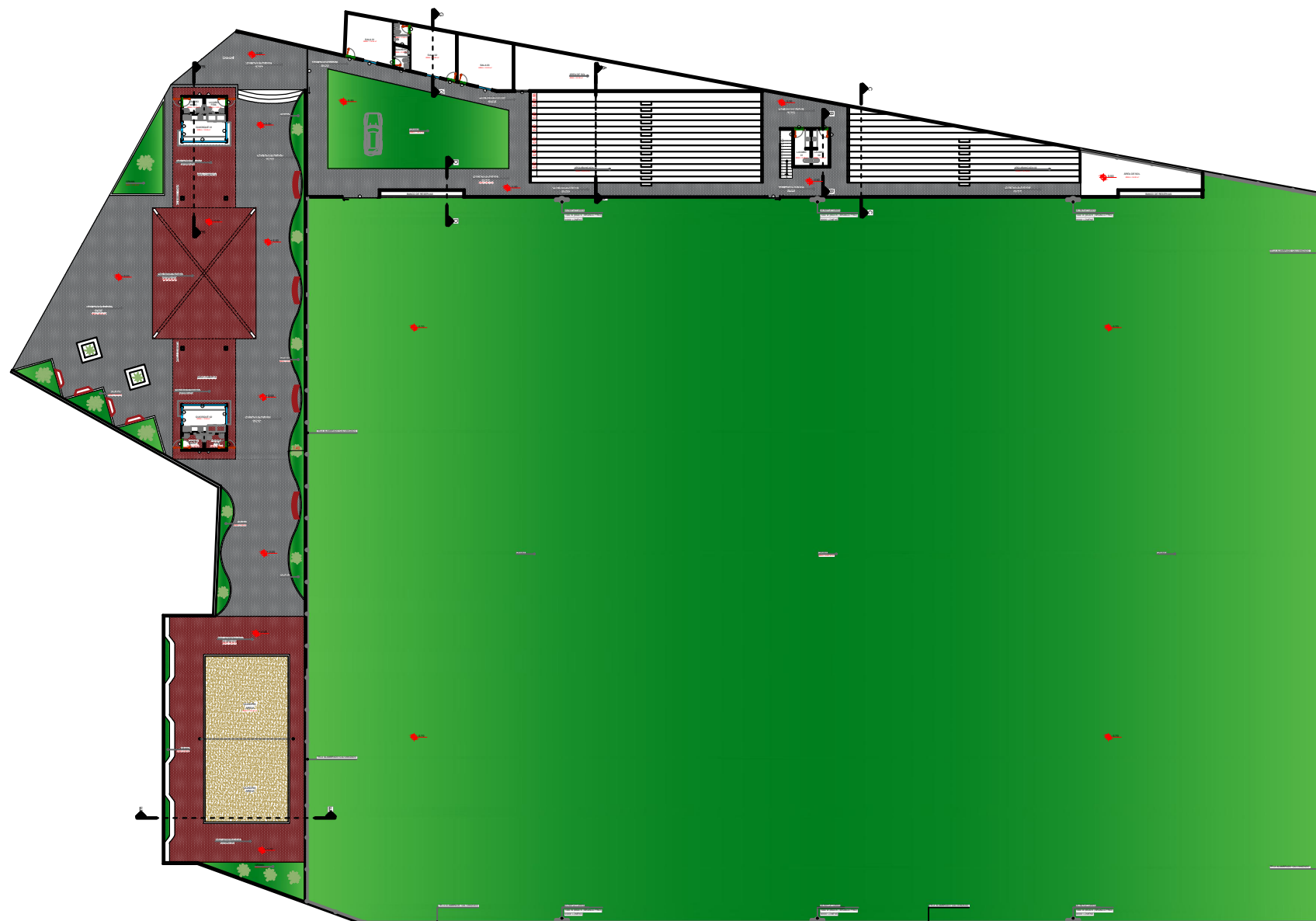
PLANTA BAIXA | IMPLANTAÇÃO ESCALA _____ 1/400
